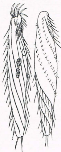
Fig. 93. Strongylidium polystichum , vtr. und dors.
