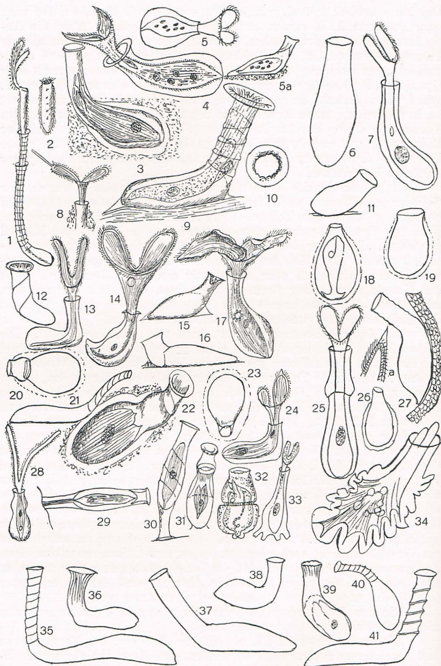
Fig. 77, 1—41 (die Größenangaben beziehen sich auf die Gehäuse).
