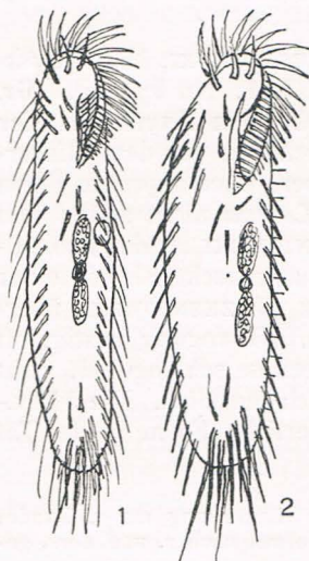
Fig. 119, 1, 2. 1 Opisthotricha sphagni . 2 O. halophila , S. 611.
