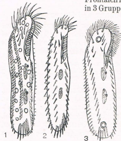
Fig. 112, 1, 2, 3. 1 Amphisiella annulata . 2 A. thiophaga . 3 A. milnei .
