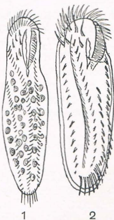
Fig. 111, 1, 2. 1 Amphisiella marioni (GOURR. u. R.). 2 Holosticha lacazei (MAUPAS). S. 579.
